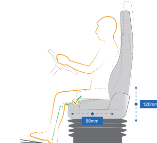
Erweiterte pneumatische Höhen- einstellung (120 mm) und Sitzkissen- tiefeinstellung (80 mm) Advanced pneu- matic height adjustment (120 mm) and seat cushion depth adjustment (80 mm)
